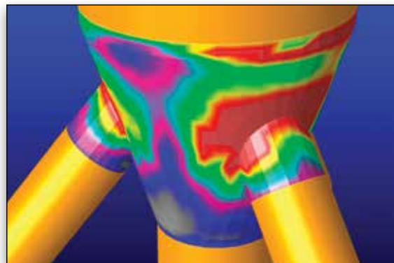
风机基础过渡段的疲劳设计参数化研究
