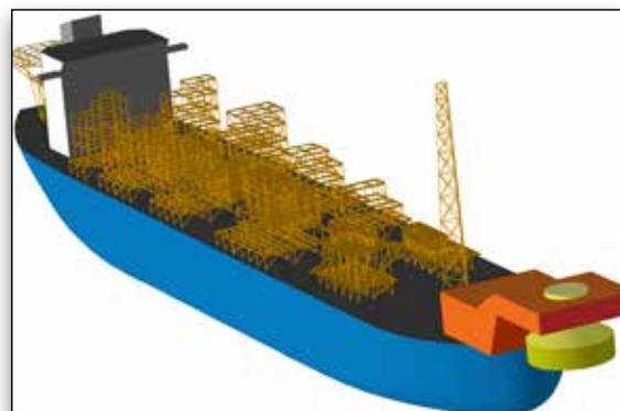
与 MOSES 进行数据交换用于 FPSO 上部结构分析
