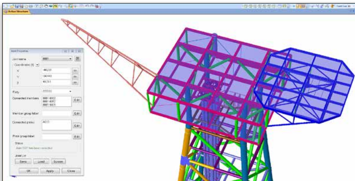
Precede Graphical Modeler 用于导管架和复杂上部结构的建模
