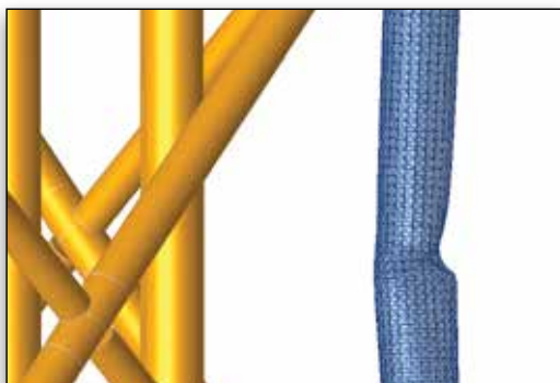
船舶撞击分析
